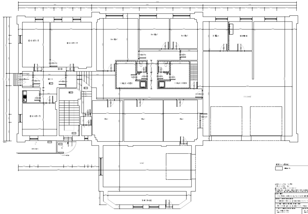
Půdorys 1.NP objektu VS Rýmařov
